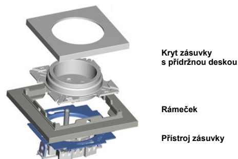
Obr. 10: Sestavování zásuvky Neo® s krytem a rámečkem
