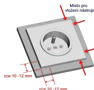
Obr. 11: Demontáž zásuvky Neo®
