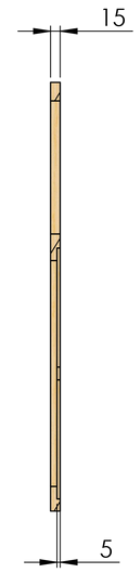
SECTION A-A
